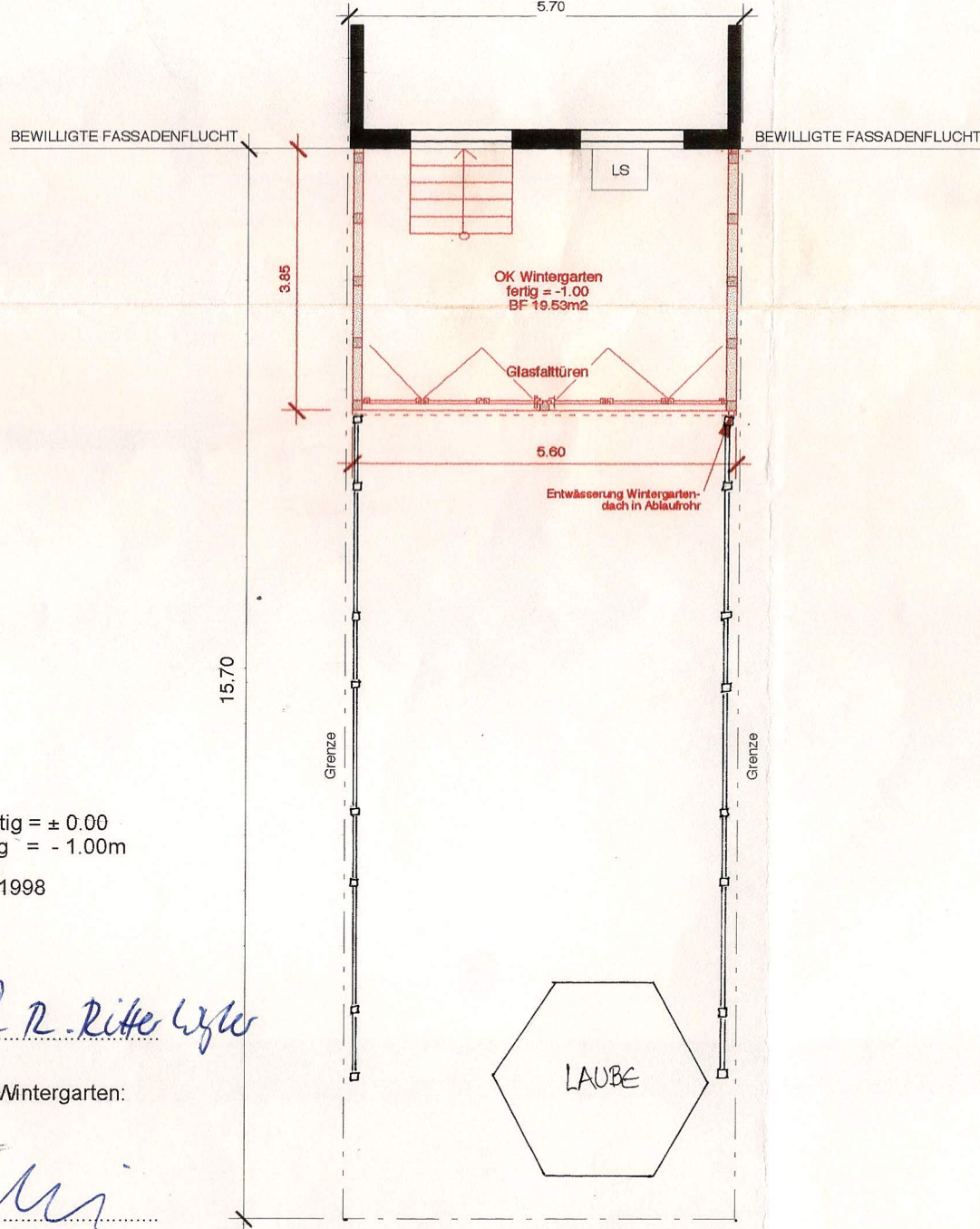
GRUNDRISS 1:100
