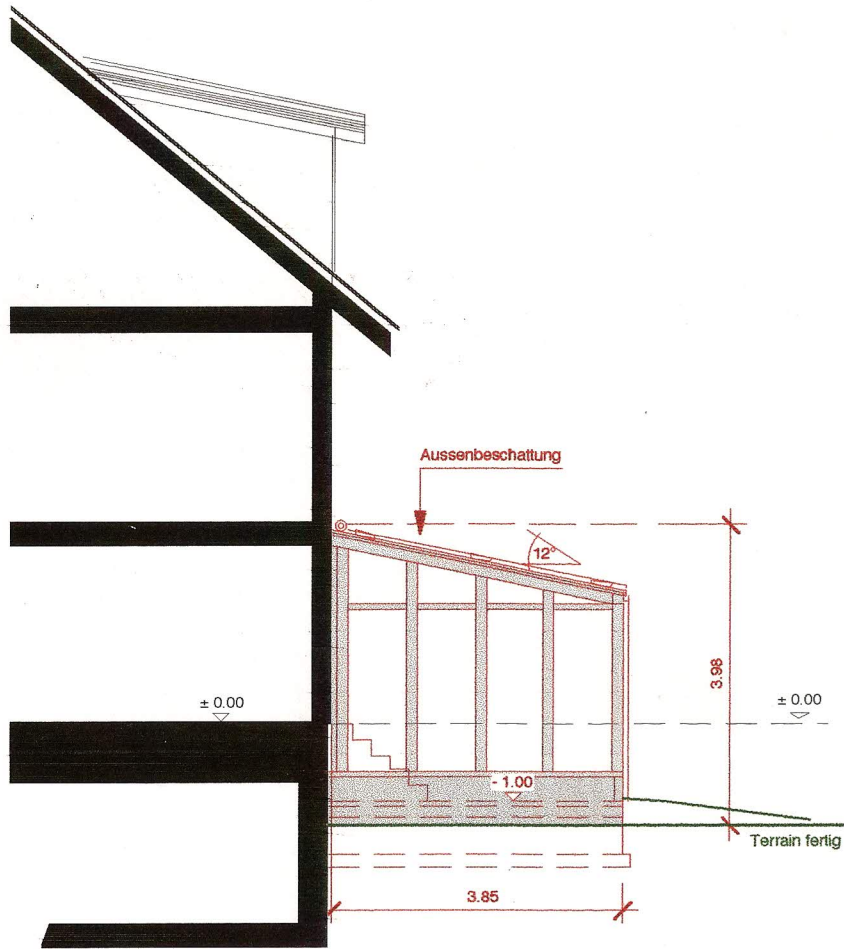
FASSADE WEST 1:100
