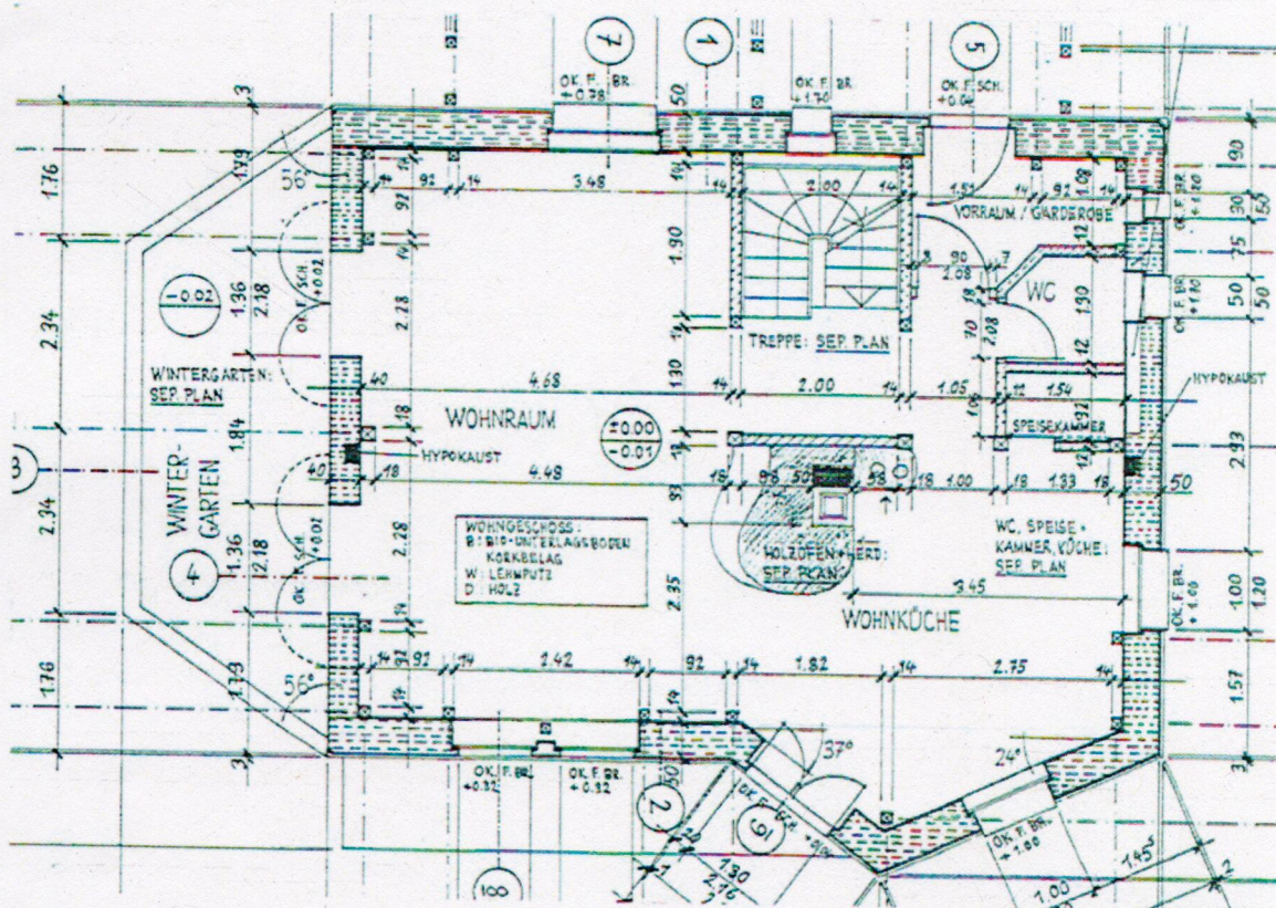
Grundriss Erdgeschoss, 1 : 100
