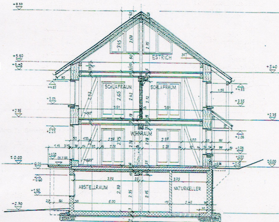
Schnitt A-A, 1 : 100
