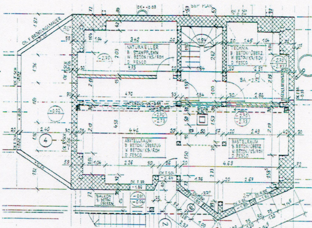
Grundriss Untergeschoss, 1 : 100
